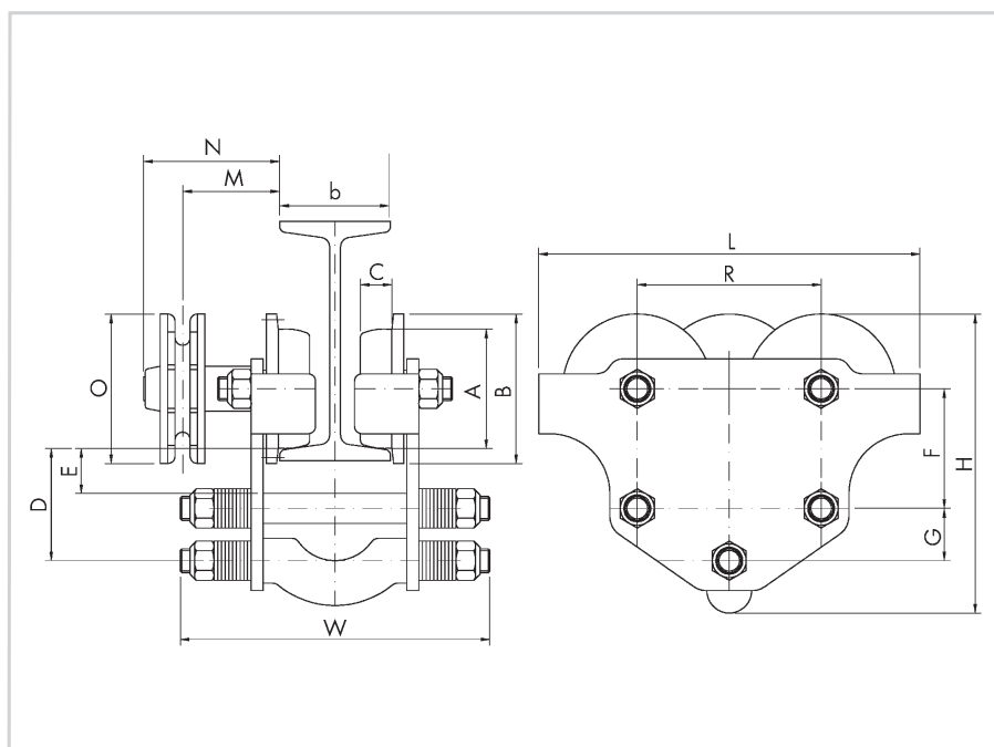
Rollfahrwerk RFW-V
